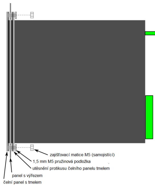
Obrázek 7.9-13 Instalace IED AQ-2xx
