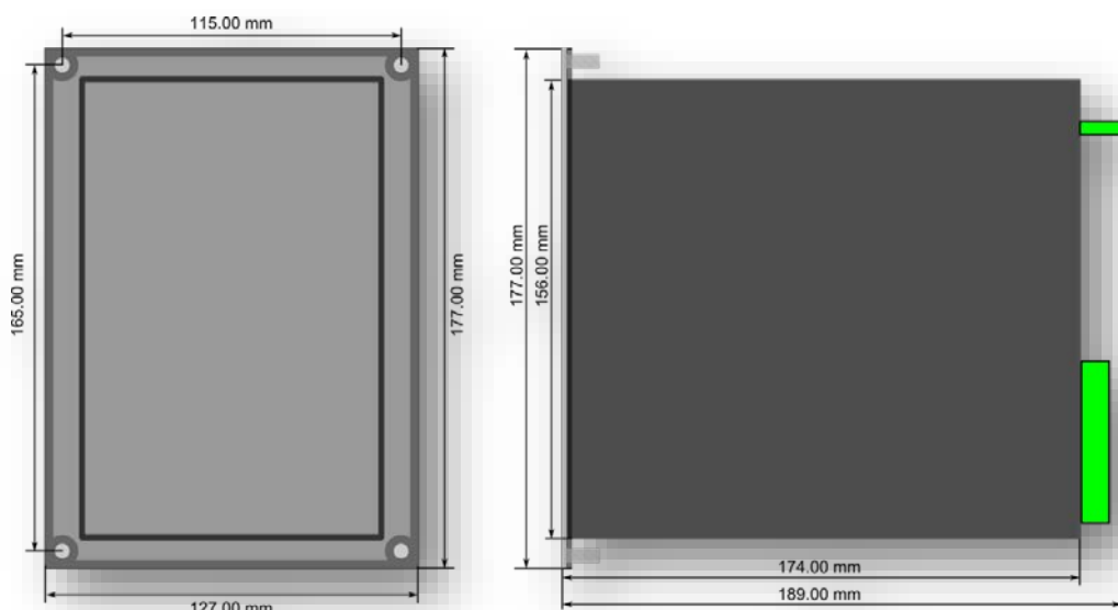
Obrázek 7.9-12 Rozměry IED AQ-2xx.
