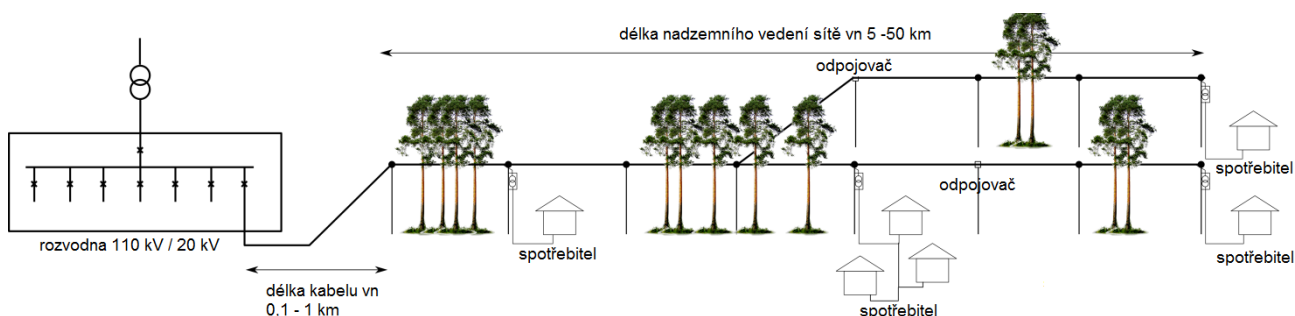
Obrázek 4.3.4.2-55 Typické uspořádání venkovské radiální sítě vysokého napětí.
