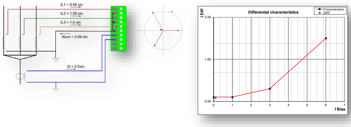
Obrázek 4.2.7.3-26 Rozdílová ochrana kabelové koncovky s přirozenou nesymetrií v měření fázových proudů.
