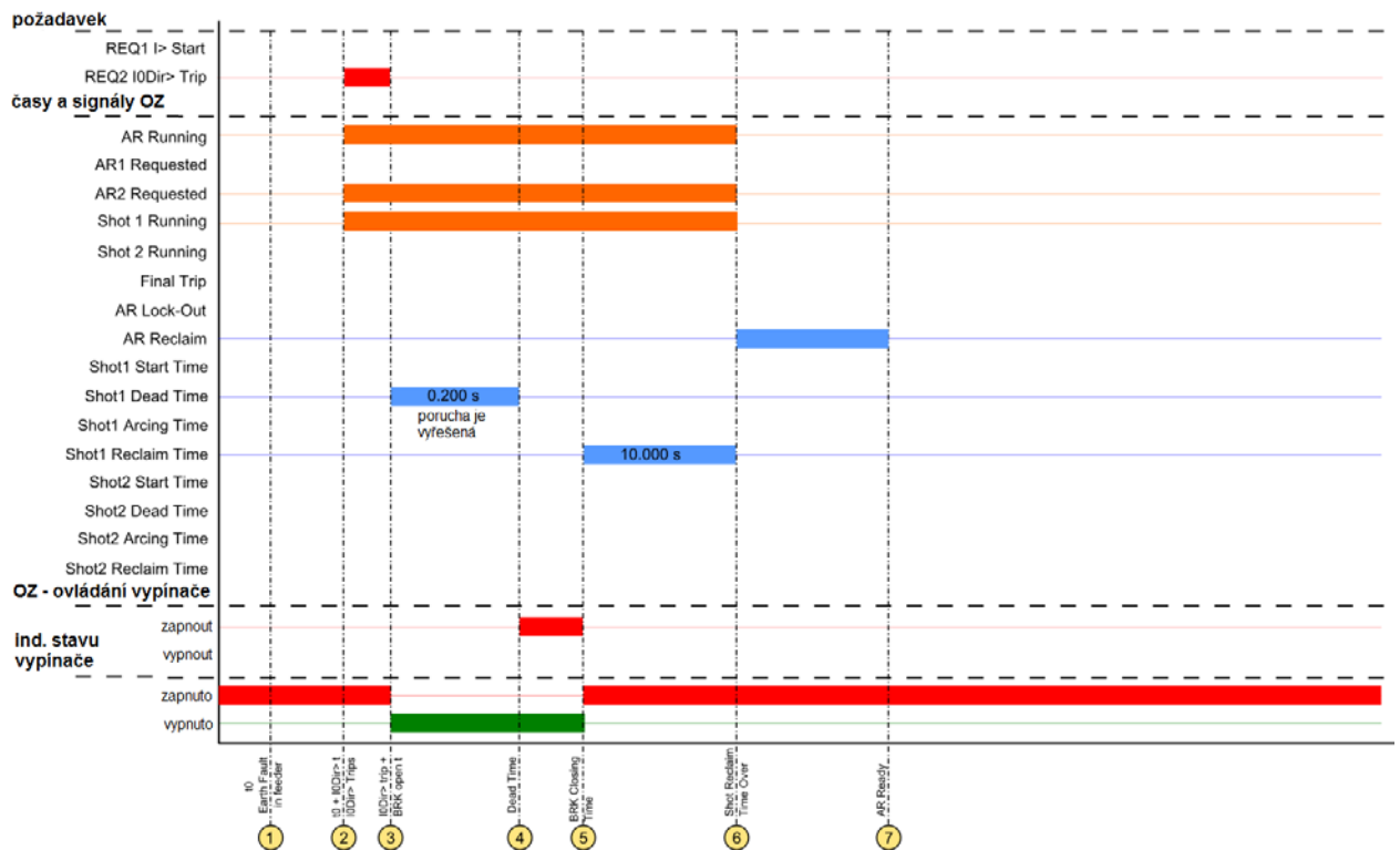
Obrázek 4.3.4.5-63 Graf stavu signálů cyklu opětného zapnutí při přechodné zemní poruše.
