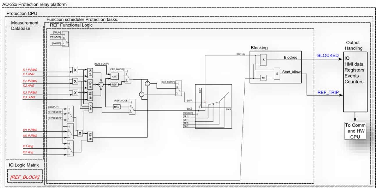
Obrázek 4.2.7-24 Zjednodušené funkční blokové schéma funkce REF.
