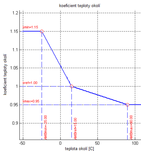
Obrázek 4.2.8-31 Příklad výpočtu koeficientu teploty okolí, pokud je referenční teplota +15 C se 3 body lineární aproximace a nastavitelnou korekční křivkou.
