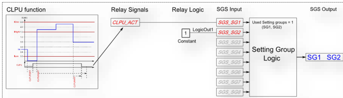
Obrázek 4.3.1.3-52 Příklad nastavení výchozího konstantního signálu SG.
