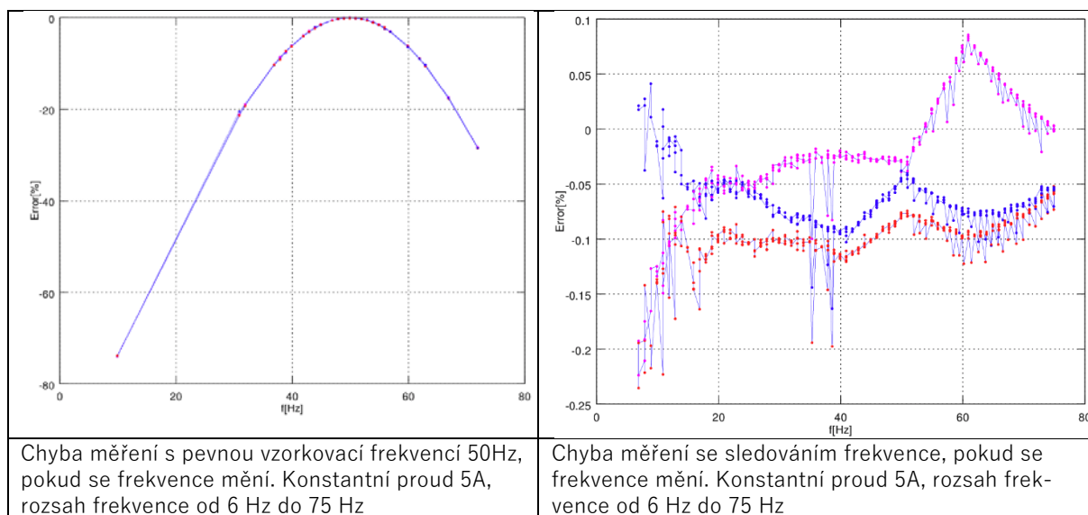
Obrázek 4.1.2-12 Efekt sledování frekvence, pokud se základní frekvence mění od 6 Hz do 75 Hz.
