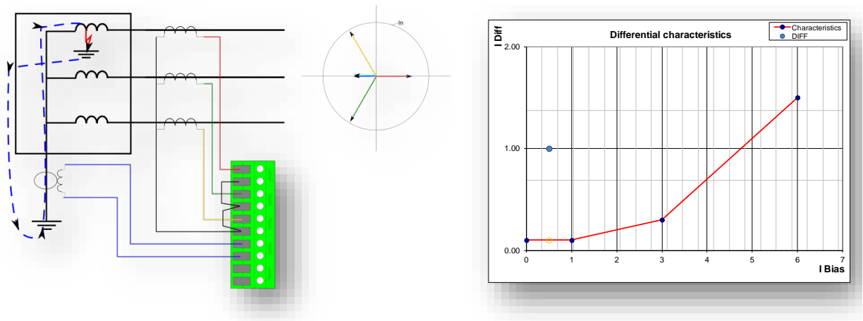
Obrázek 4.2.7.3-29 Zemní porucha na vnitřní straně vinutí transformátoru Y.
