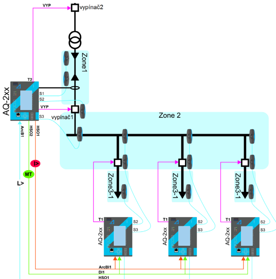
Obrázek 4.2.10-45 Schéma IA1: jednopólové schéma s relé série AQ-2xx.
