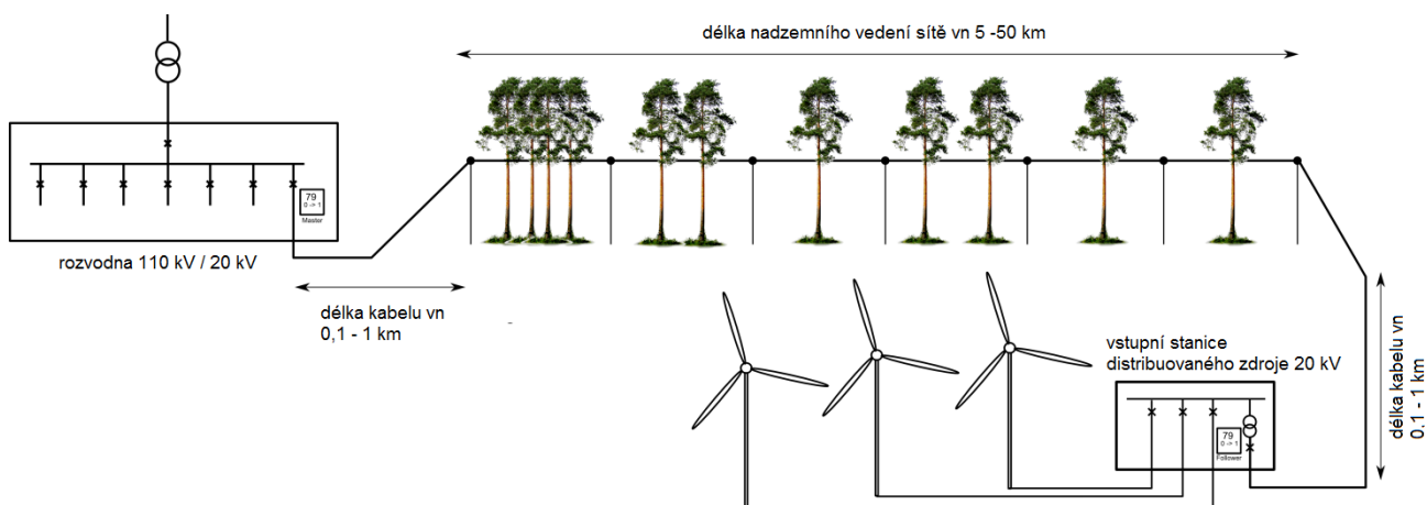
Obrázek 4.3.4.9-70 Automatika opětného zapnutí s distribuovaným zdrojem ve vedení.
