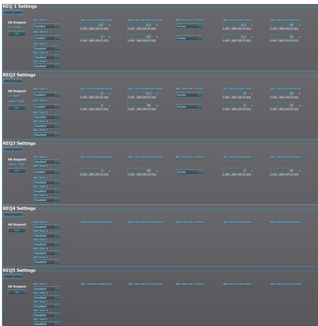
Obrázek 4.3.4.14-72 Parametry nastavení pokusu automatiky OZ.
