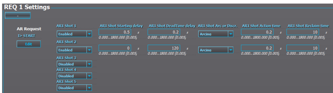
Obrázek 4.3.4.8-68 Nastavení pro opětné zapnutí při nadproudové poruše se dvěma pokusy.
