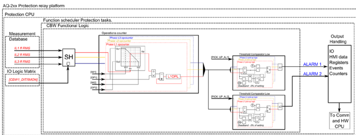
Obrázek 4.4.4-92 Zjednodušené funkční blokové schéma funkce CBW.
