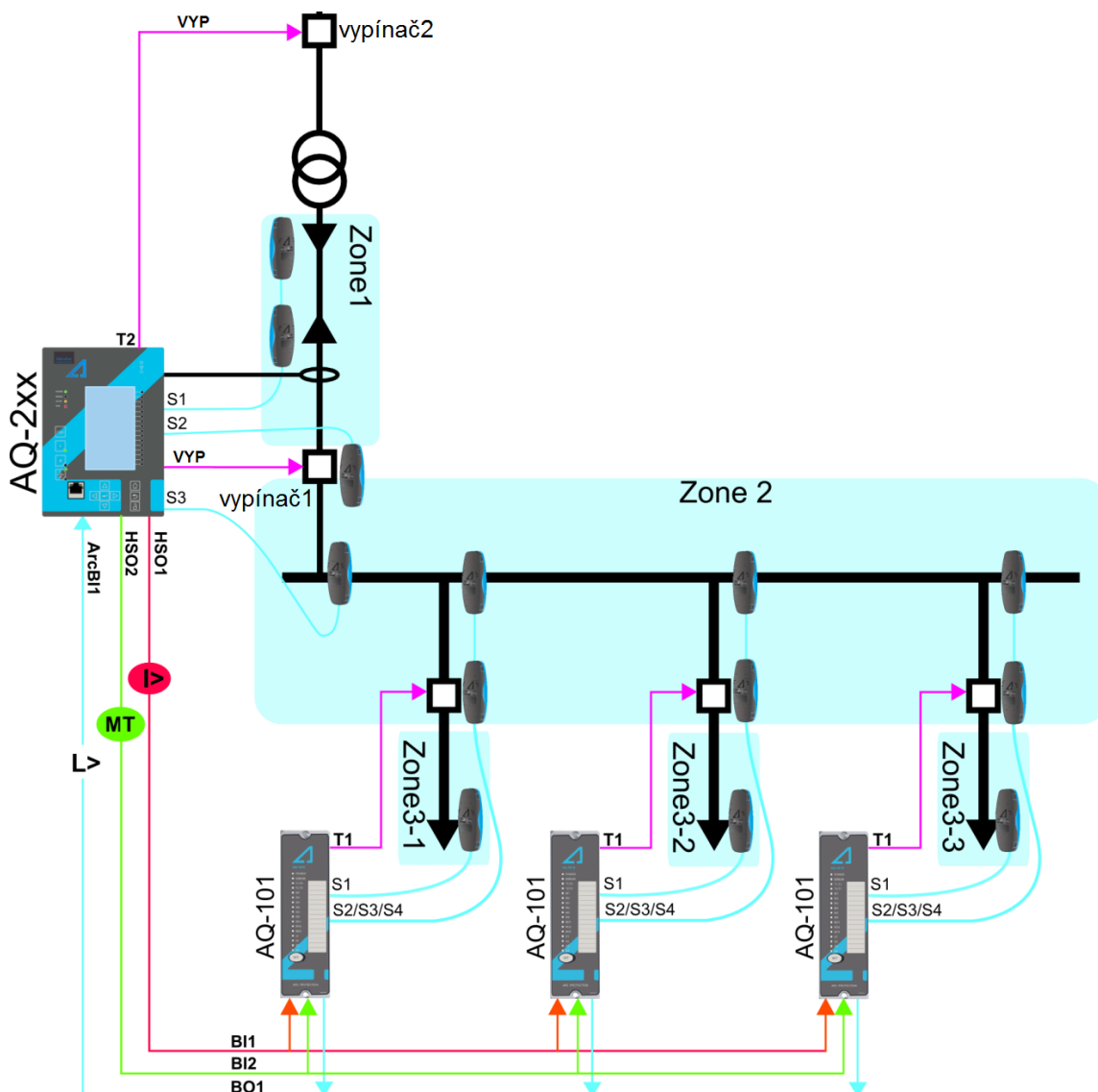
Obrázek 4.2.10-44 Schéma IA1: jednopólové schéma s relé série AQ-2xx a relé zábleskové ochrany AQ-101.
