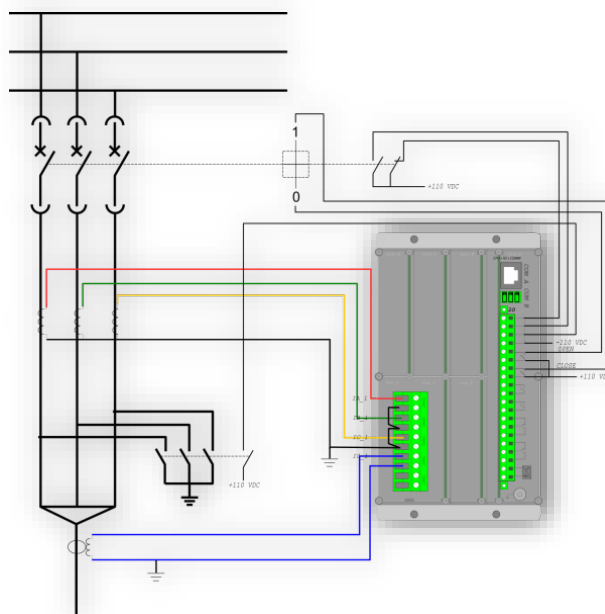
Obrázek 4.3.2.3-54 Příklad aplikace blokování. Zapnutý uzemňovač blokuje zapnutí vypínače.
