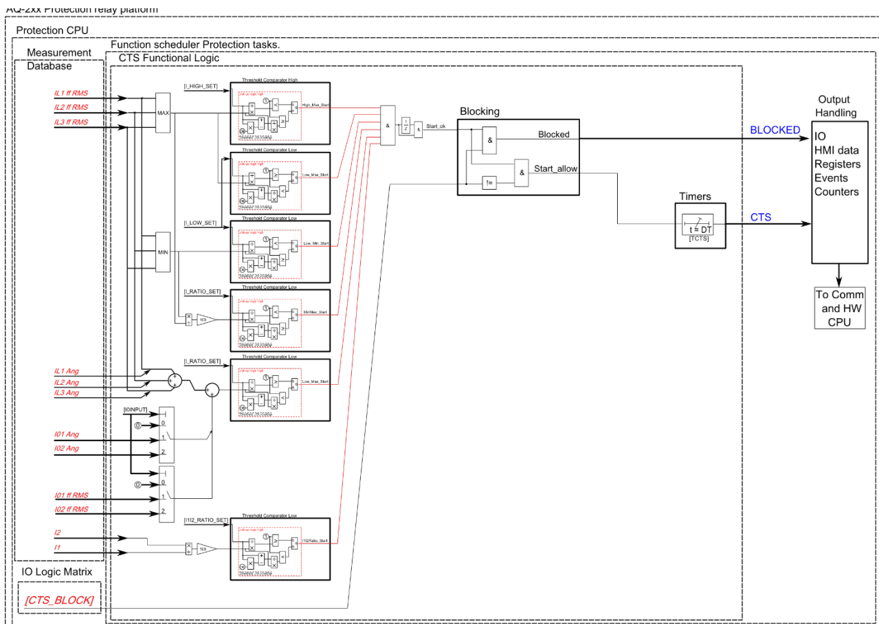
Obrázek 4.4.1-81 Zjednodušené funkční blokové schéma funkce CTS.
