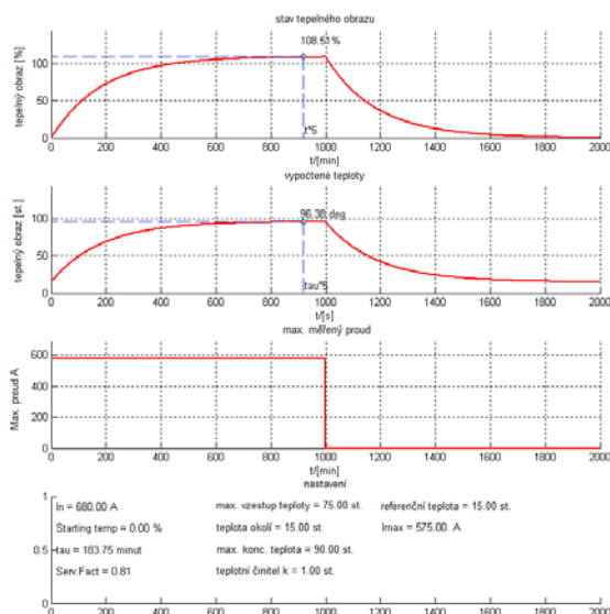
Obrázek 4.2.8-40 Reakce tepelného obrazu s jmenovitým proudem a přesně vyladěným korekčním činitelem k_{SF} .
