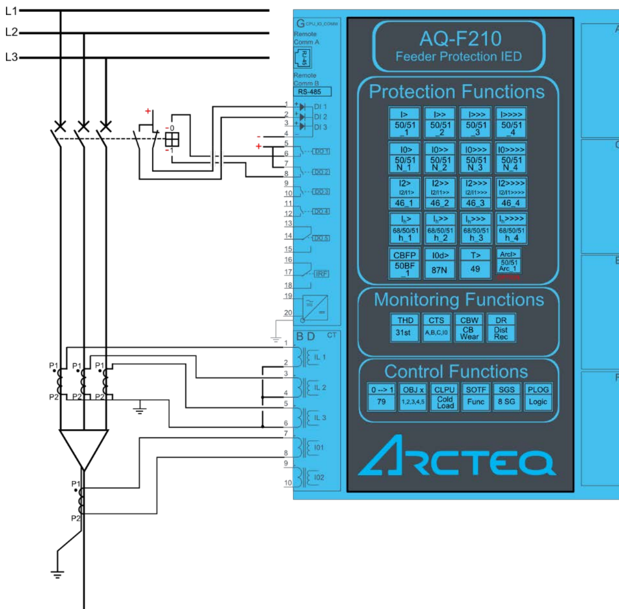
Obrázek 8.2-1 Příklad zapojení AQ-F210
