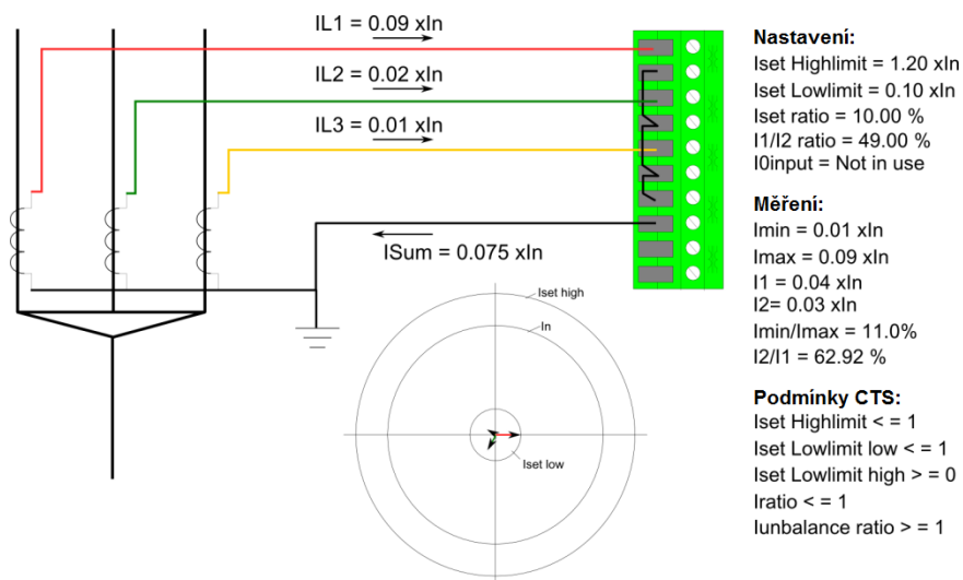
Obrázek 4.4.1.5-86 Systém v případě malého proudu a velké nesymetrie.
