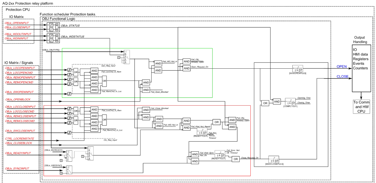
Obrázek 4.3.2-53 Zjednodušené funkční blokové schéma funkce OBJ.
