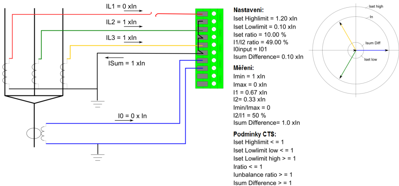
Obrázek 4.4.1.5-88 Systém v případě přerušení sekundárního fázového proudu.
