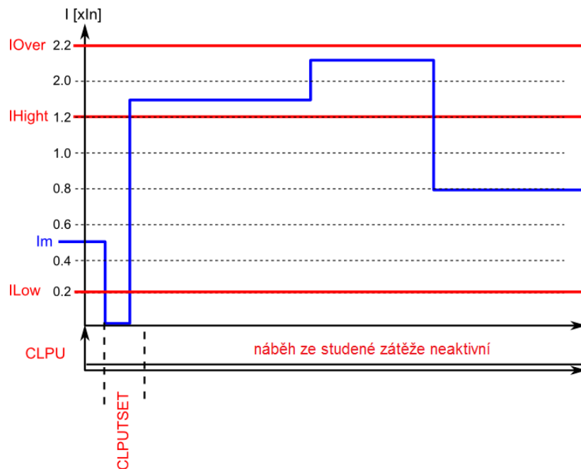
Obrázek 4.3.5.4-75 Příklad parametrů pro časy a náběh. Bez náběhu CLPU pro krátkou dobu nízkého proudu.
