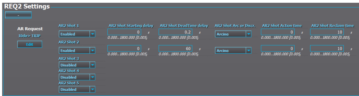
Obrázek 4.3.4.5-62 Nastavení pro opětne zapnutí při zemní poruše se dvěma pokusy.
