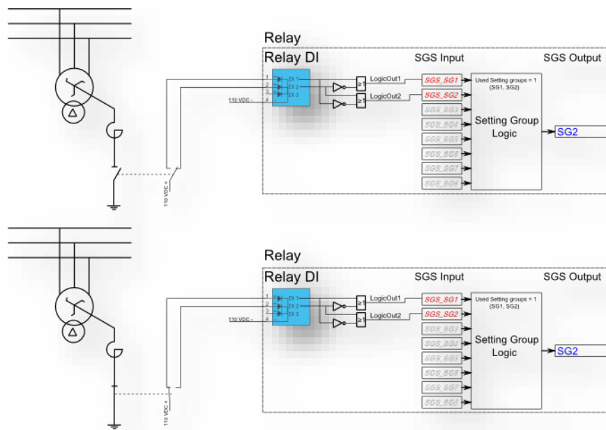
Obrázek 4.3.1.3-50 Ovládání skupiny nastavení s připojením stavu Petersenovy tlumivky dvěma vodiči a přidavnou logikou.
