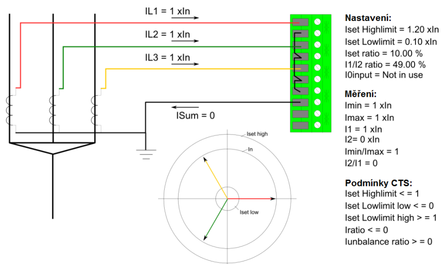
Obrázek 4.4.1.5-82 Systém v případě, že vše funguje správně a neexistuje žádná porucha.
