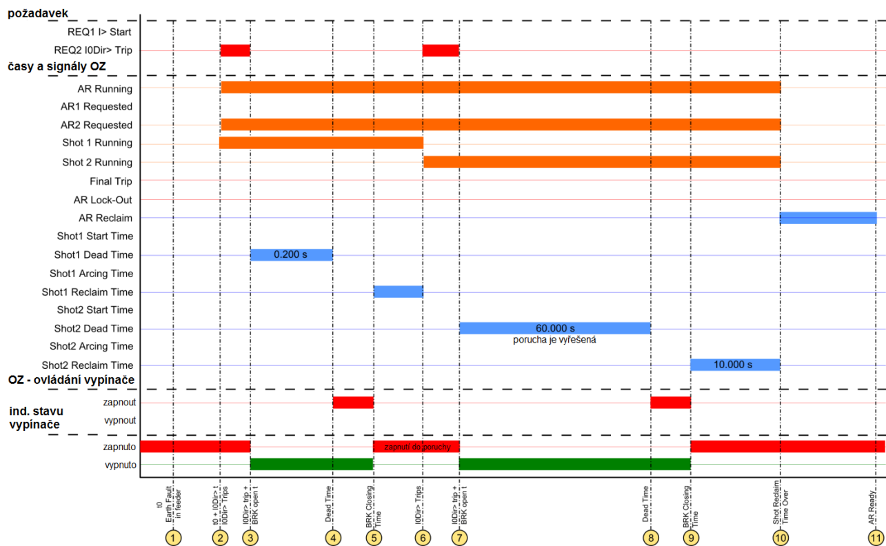
Obrázek 4.3.4.4-61 Graf stavu signálů cyklu opětného zapnutí při částečné zemní poruše.
