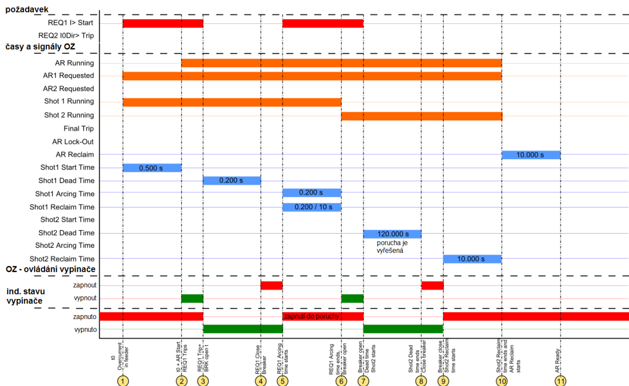
Obrázek 4.3.4.7-67 Graf stavu signálů cyklu opětného zapnutí při částečné nadproudové poruše.
