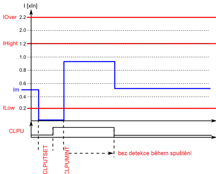
Obrázek 4.3.5.4-78 Příklad parametrů pro časy a náběh. Během spuštění není detekován zapínací proud.
