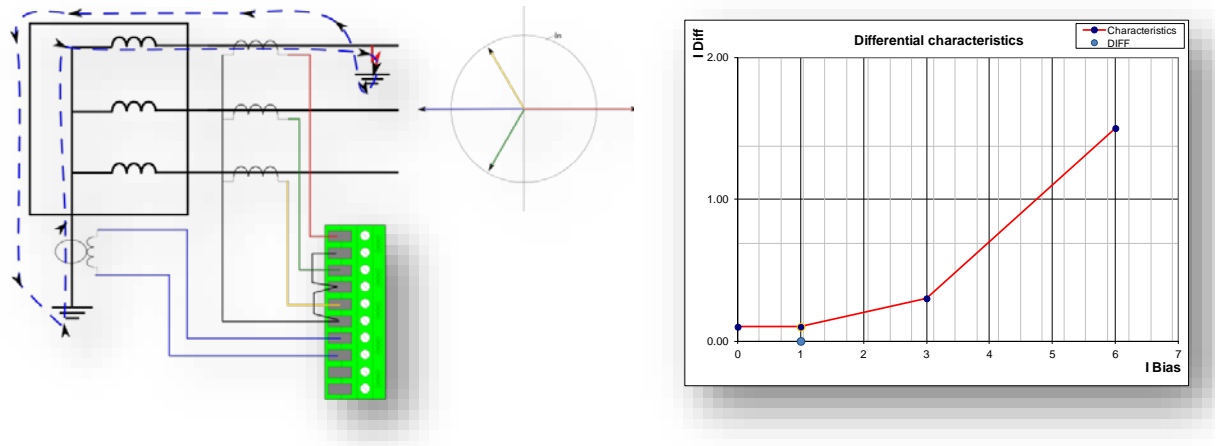
Obrázek 4.2.7.3-28 Zemní porucha na vnější straně vinutí transformátoru Y.
