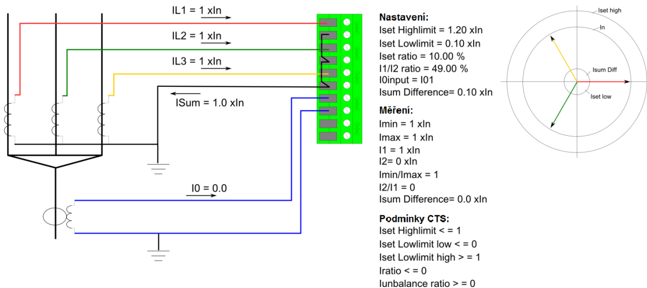
Obrázek 4.4.1.5-87 Systém v normální stavu s měřením zemního proudu.
