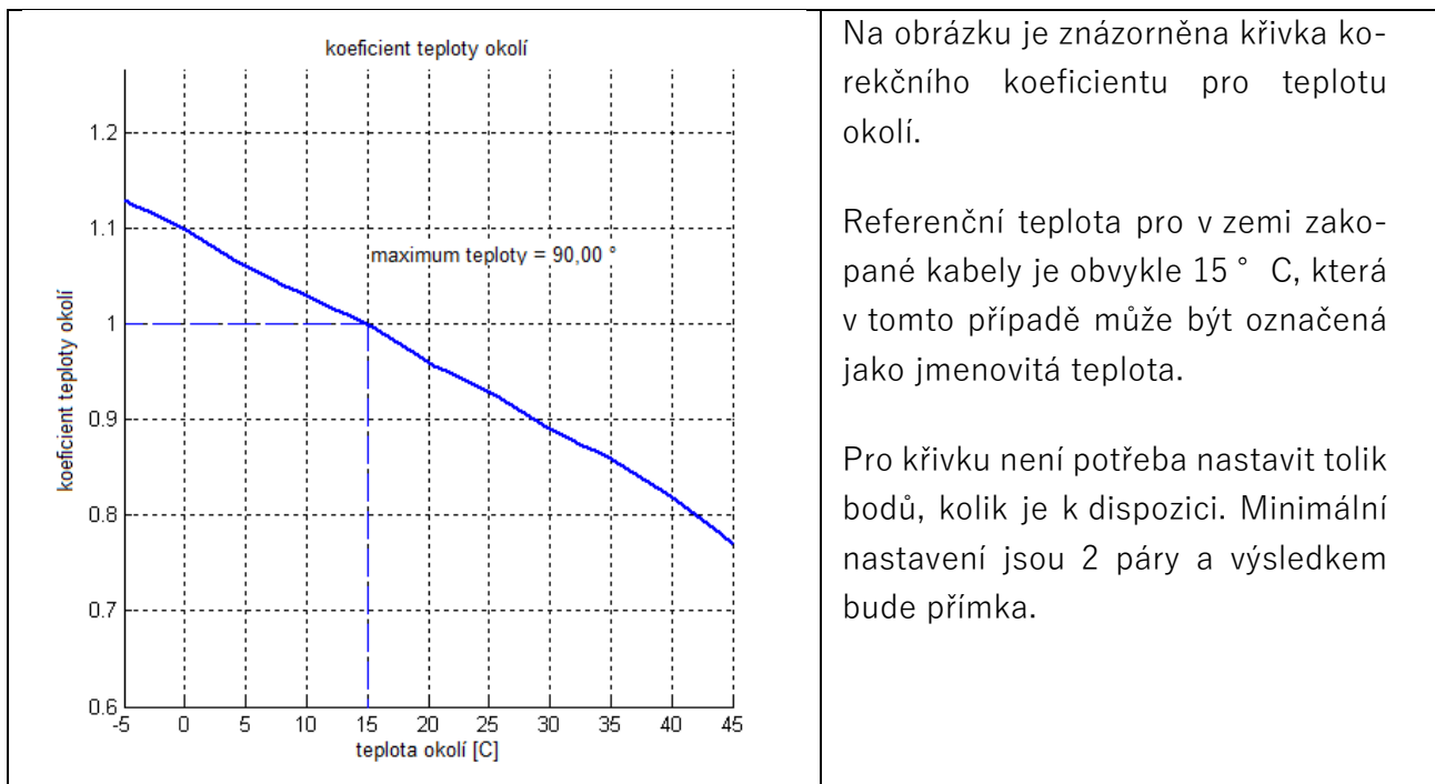
Obrázek 4.2.8-34 Nastavení korekční křivky pro teplotu okolí.
