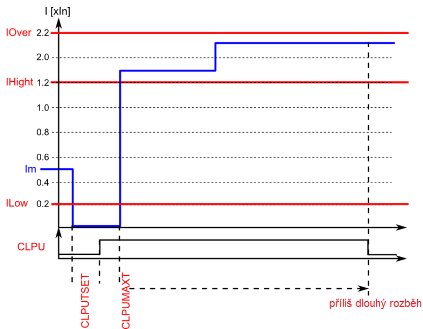
Obrázek 4.3.5.4-77 Příklad parametrů pro časy a náběh. Během spuštění není detekován zapínací proud.
