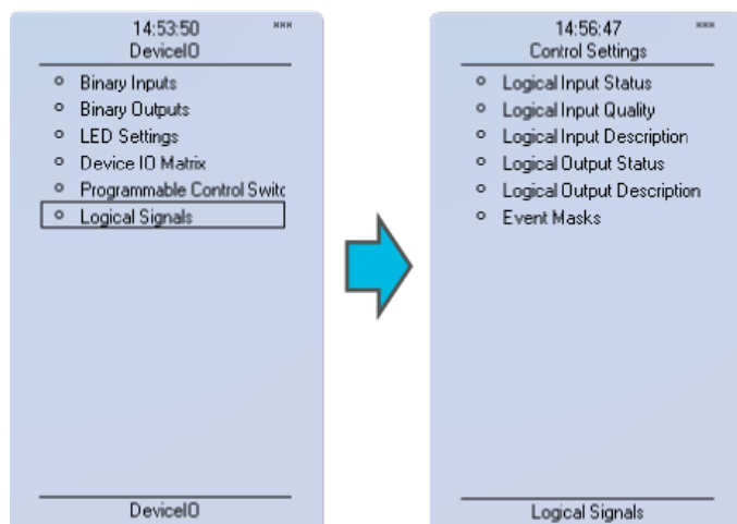
Obrázek 3.1.2.3-28 Logické signály IED série AQ-200.
