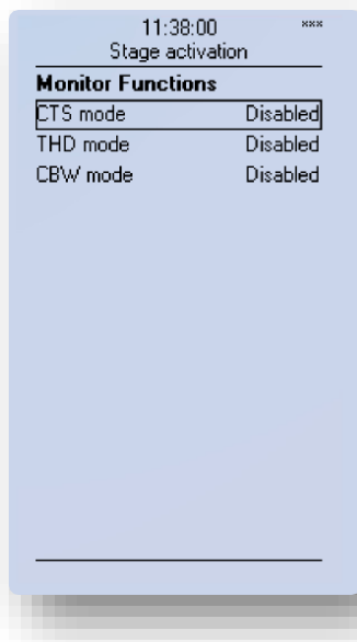
Obrázek 3.1.2.6-38 Podmenu pro povolení monitorování IED série AQ-200.
