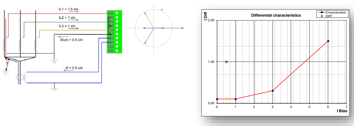
Obrázek 4.2.7.3-27 Rozdílová ochrana kabelové koncovky při vzniku poruchy.
