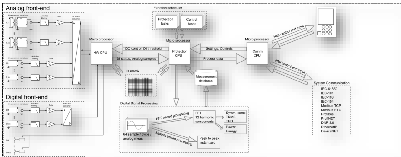
Obrázek 4.2.1-13 Principiální schéma platformy ochrany AQ-2xx.
