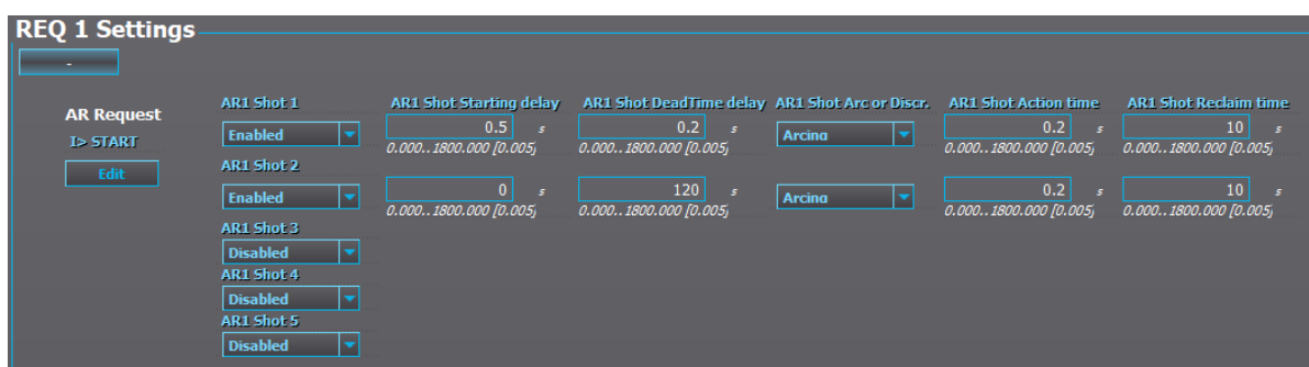
Obrázek 4.3.4.6-64 Nastavení pro opětné zapnutí při nadproudové poruše se dvěma pokusy.
