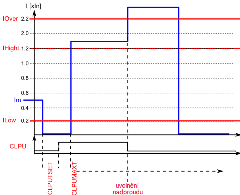
Obrázek 4.3.5.4-76 Příklad parametrů pro časy a náběh. Okamžité uvolnění aktivovaného CLPU kvůli příliš dlouhému rozběhu.
