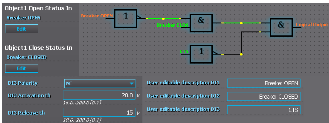
Obrázek 8.3.2-7 Blokové schéma kontroly vyp. obvodu, pokud se nepoužívá vypínací výstup bez přidrž.
