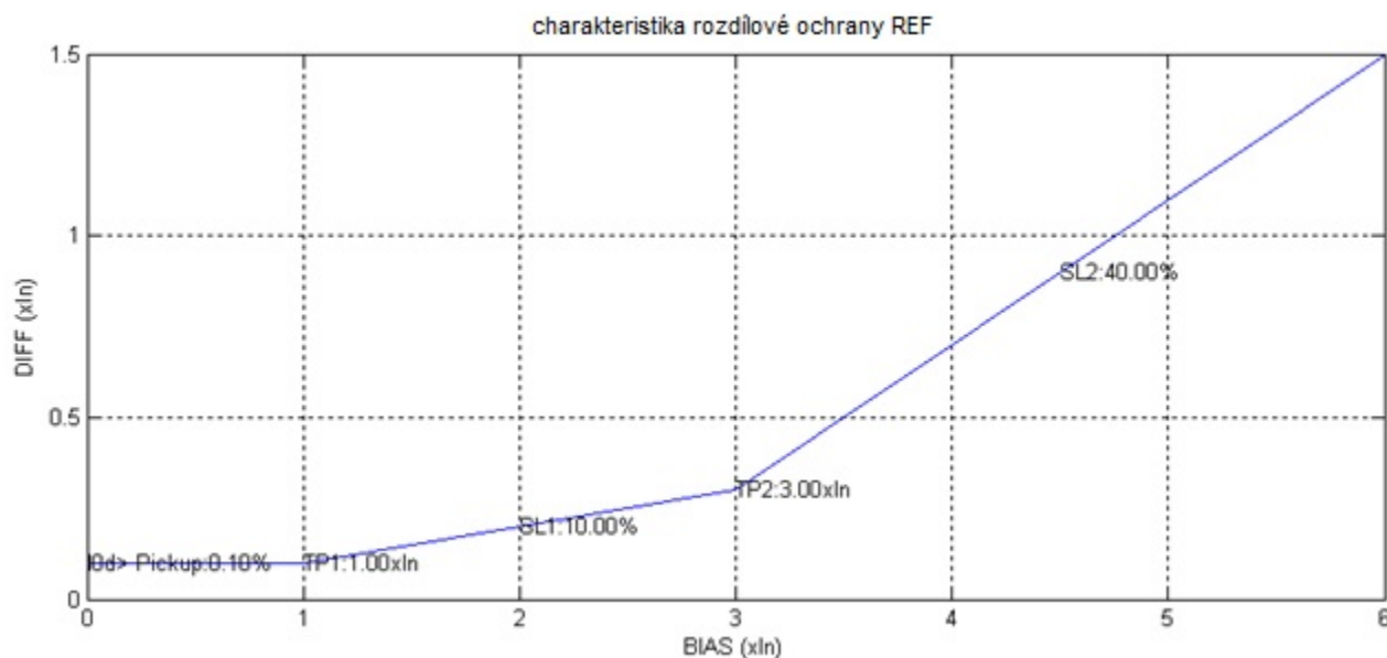
Obrázek 4.2.7.2-25 Rozdílová charakteristika pro funkci REF s výchozím nastavením.
