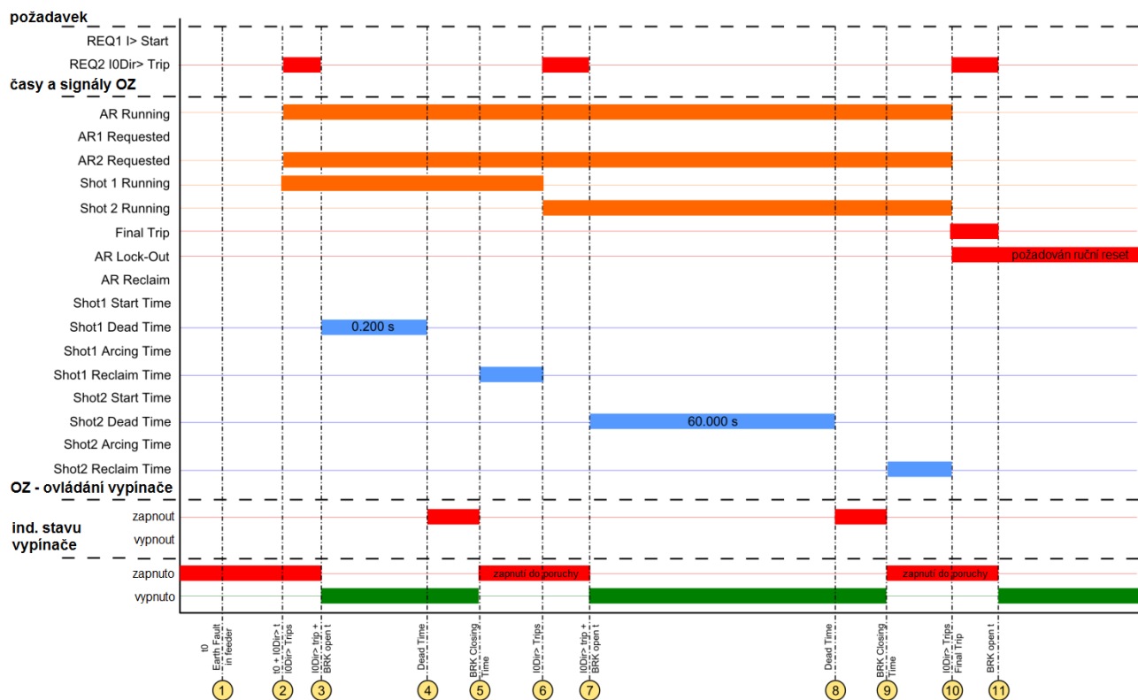
Obrázek 4.3.4.3-59 Graf stavu signálů cyklu opětného zapnutí při trvalé zemní poruše.
