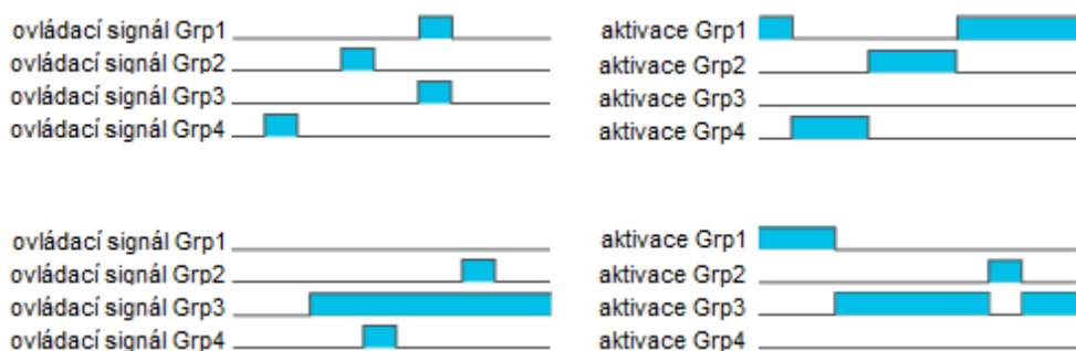
Obrázek 4.2.10.5-47 Změna skupiny jen pulzním ovládním nebo pulzem a statickým signálem.
