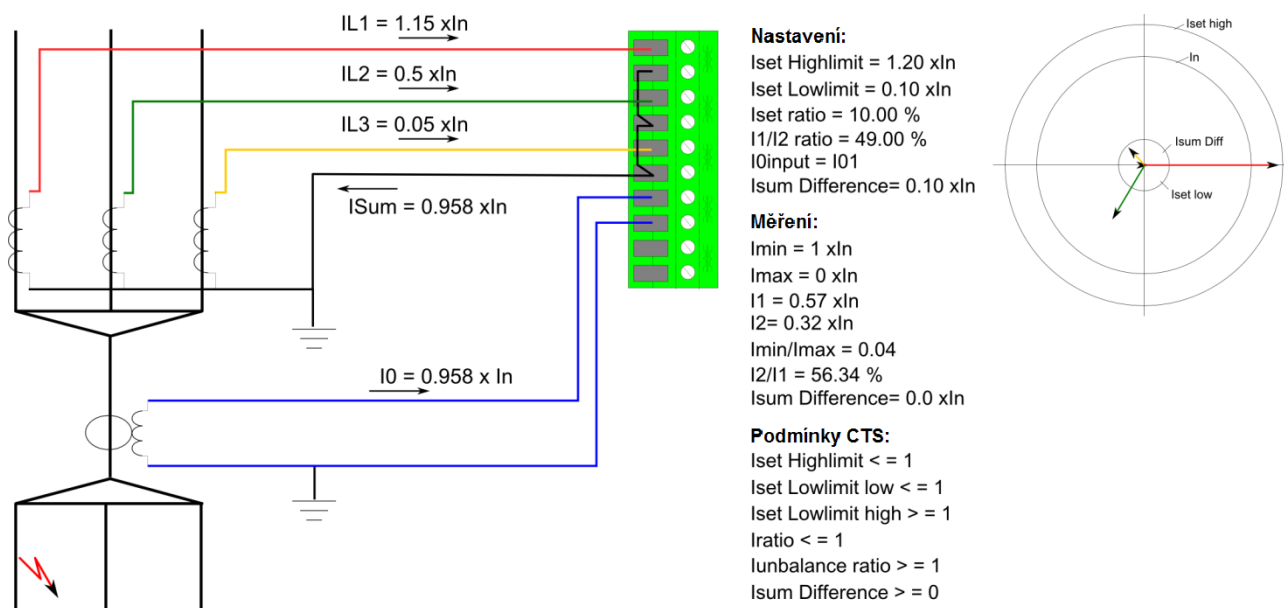
Obrázek 4.4.1.5-90 Systém v případě vysokoimpedanční zemní poruchy na primární straně.
