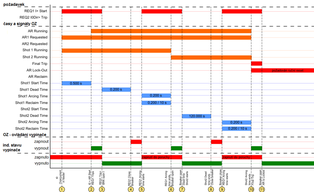
Obrázek 4.3.4.6-65 Graf stavu signálů cyklu opětného zapnutí při trvalé nadproudové poruše.
