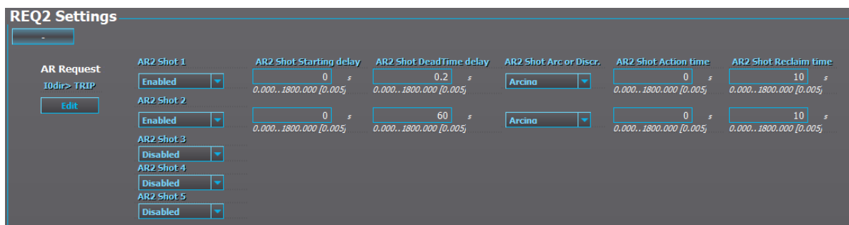
Obrázek 4.3.4.4-60 Nastavení pro opětne zapnutí při zemní poruše se dvěma pokusy.
