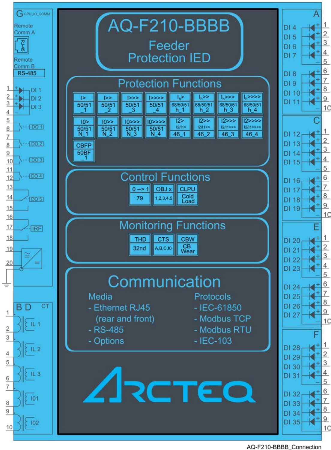
Obrázek 5.2-2 Blokové schéma varianty AQ-F210-BBBB s přidavnými moduly DI8 ve všech konfigurovatelných slotech.
