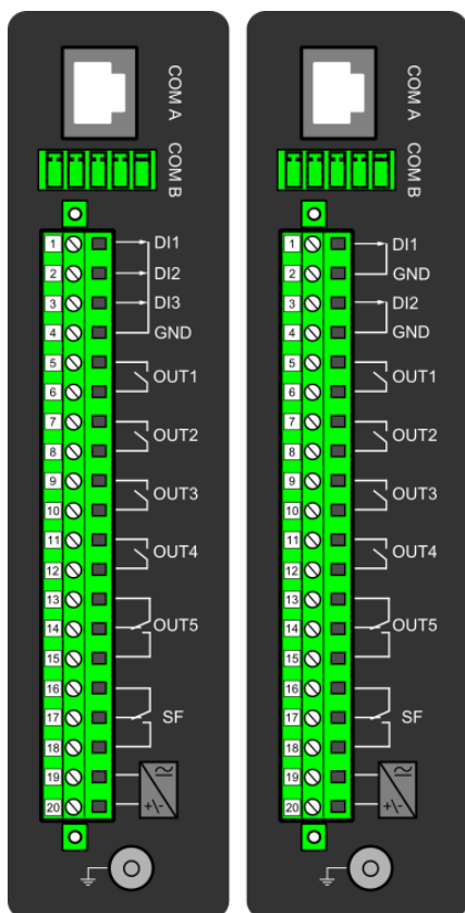
Obrázek 7.1-3 AQ-2xx Modul hlavního procesoru CPU, IO, komunikace a zdroje.
